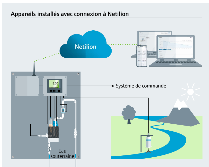
Vue d'ensemble de l'installation de Netilion au Wasserwerk Reinach und Umgebung
